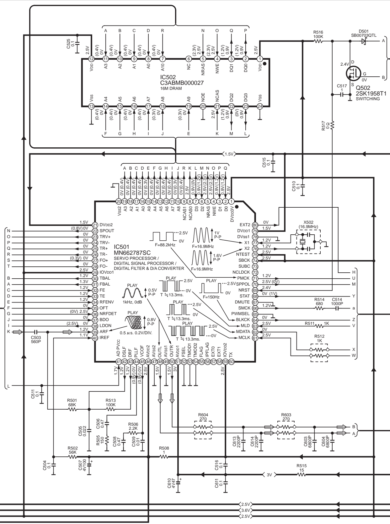
SL-CT590(EB,EG) CIRCUIT DIAGRAM
